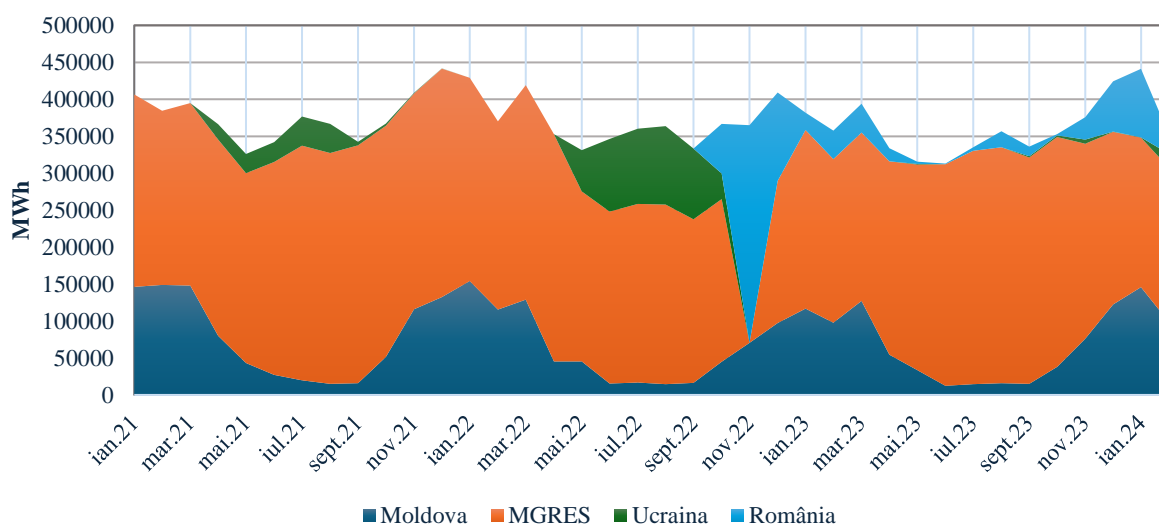
Figura 7. Consumul energiei electrice în perioada ianuarie 2021 – februarie 2024 17
